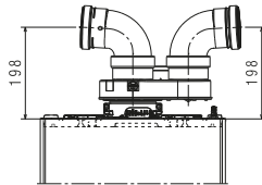
CONDOTTI SDOPPIATI Ø80-80 mm CON ADATTATORE
