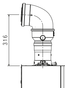
CONDOTTO COASSIALE Ø80-125 mm
