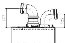
CONDOTTI SDOPPIATI Ø80-80 mm
